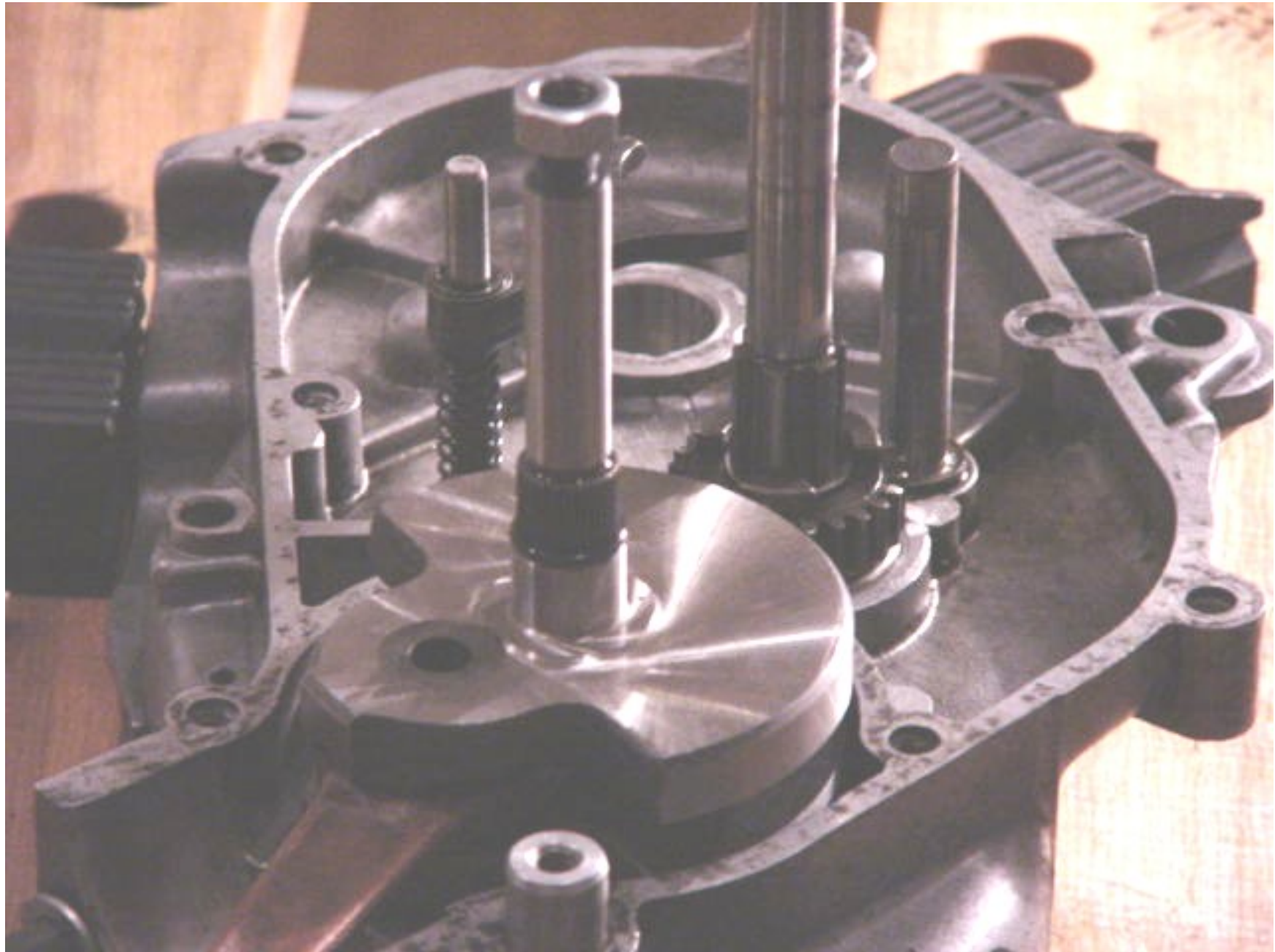
Inserting the main gear axle Seite 5 von 14
